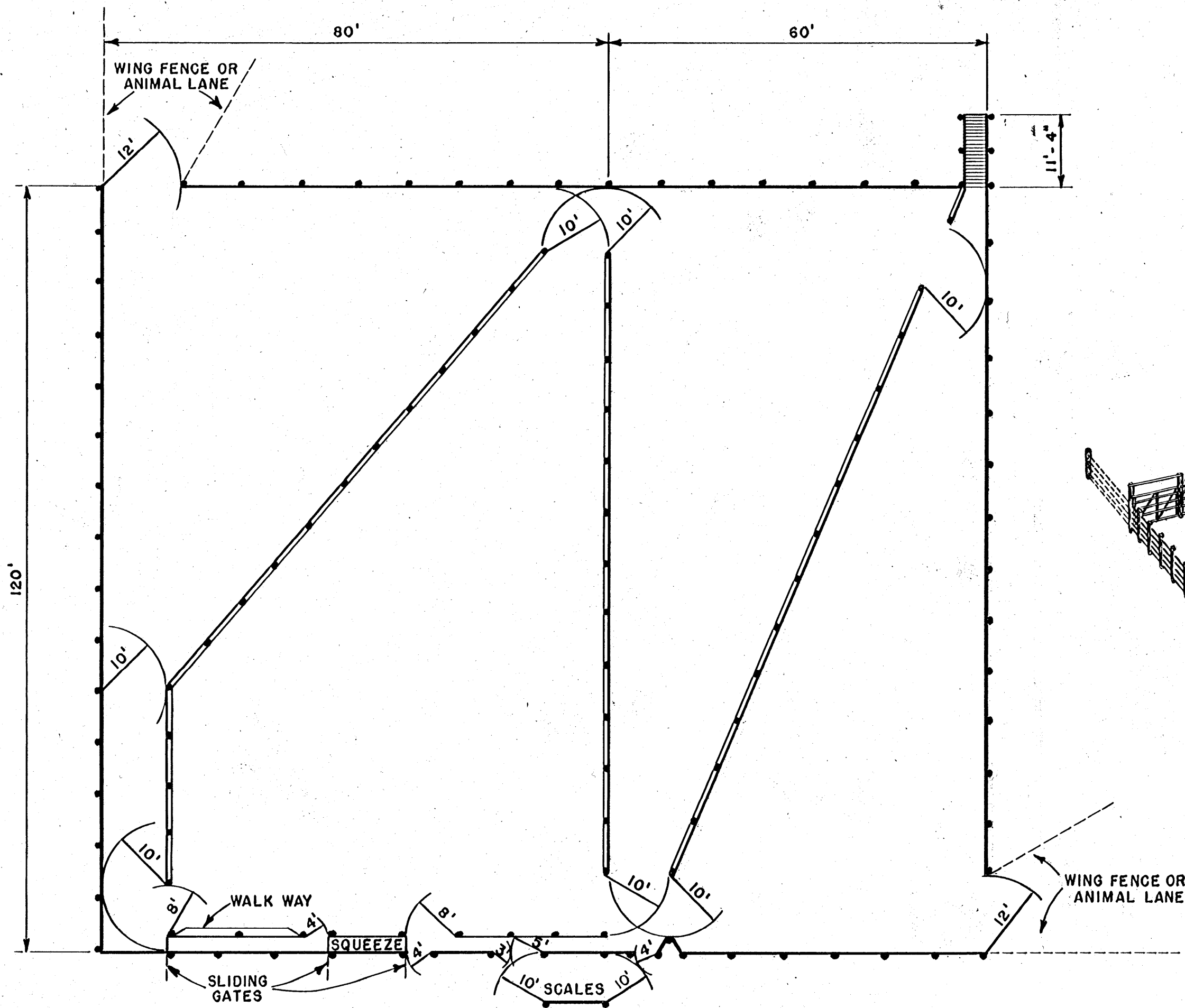
PLAN SCALE: 1/16" = 1'-0"
